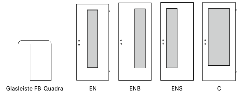
Glaslichtenausführungen:
