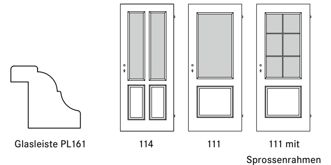
Glaslichtenausführungen:
