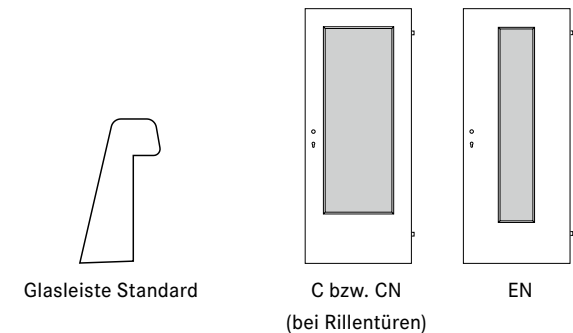
Glaslichtenausführungen:
