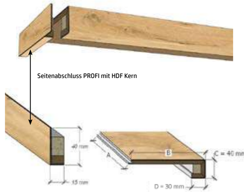
Trittstufe wird mit Bodendiele fortgeführt
